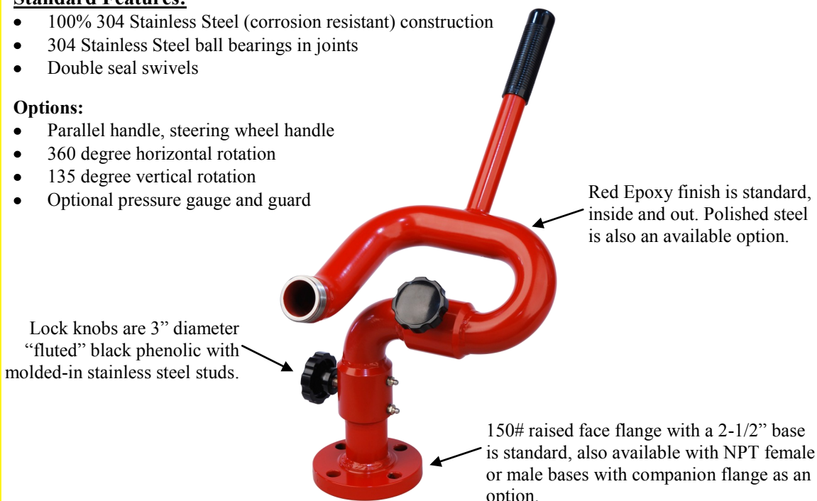
FP3S-750 SHOWN
